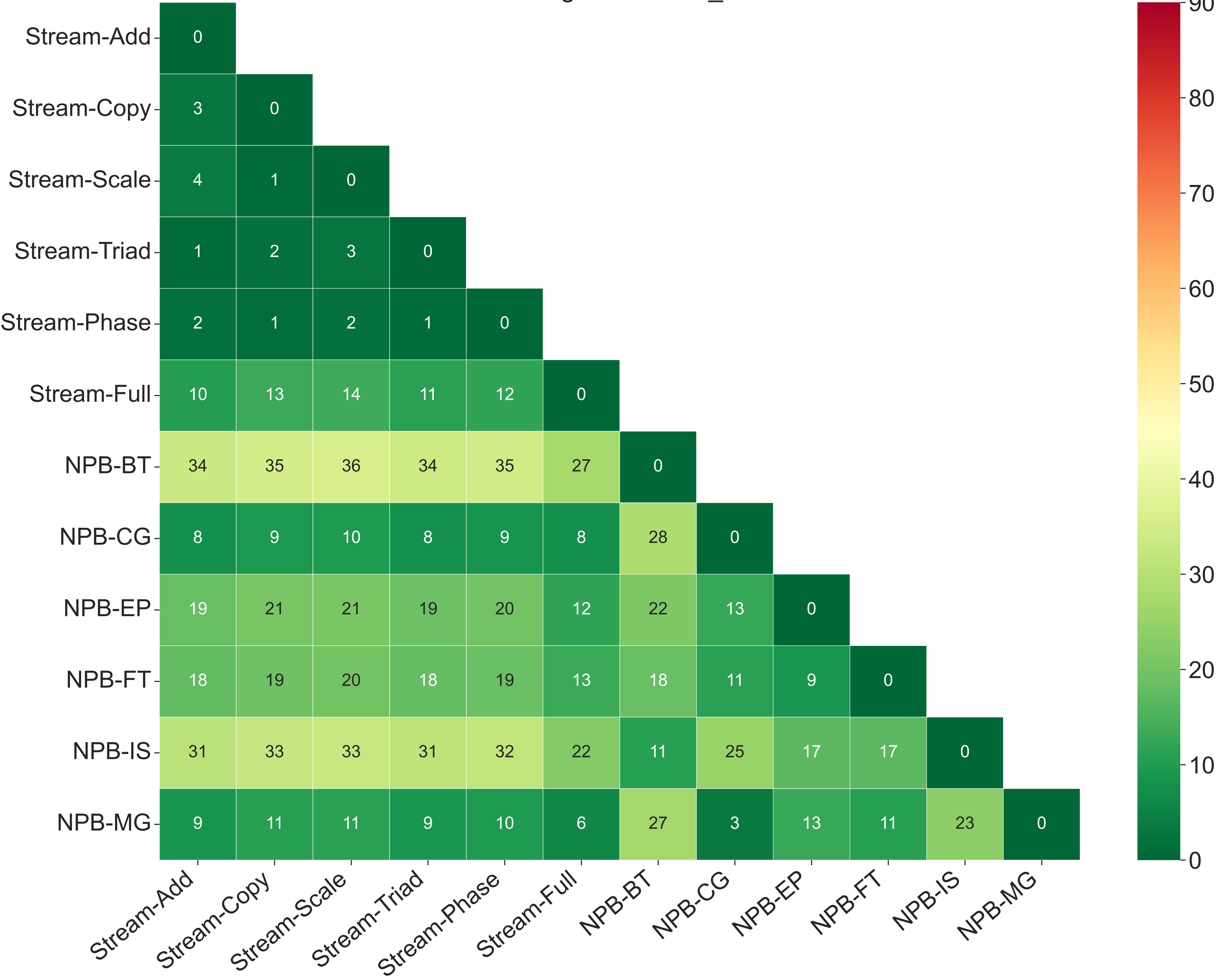
JS-divergence PCAP_89.0
