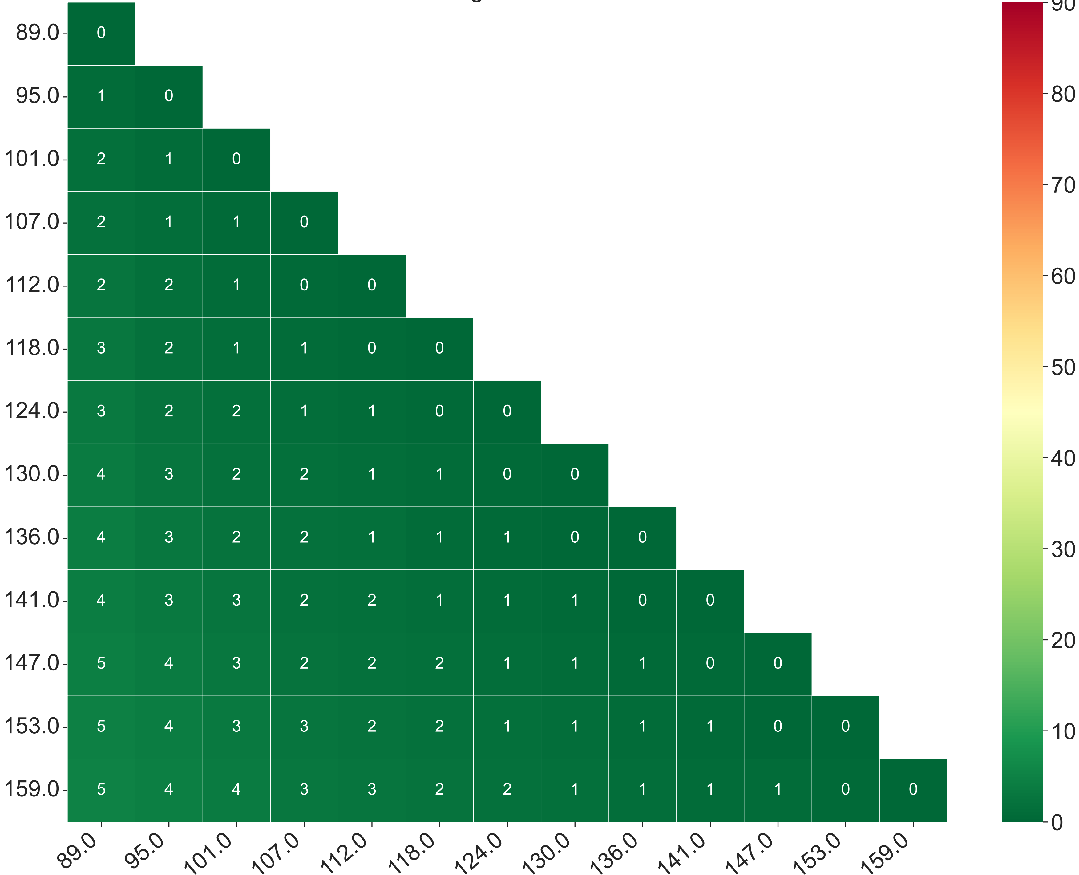
JS-divergence NPB-BT
