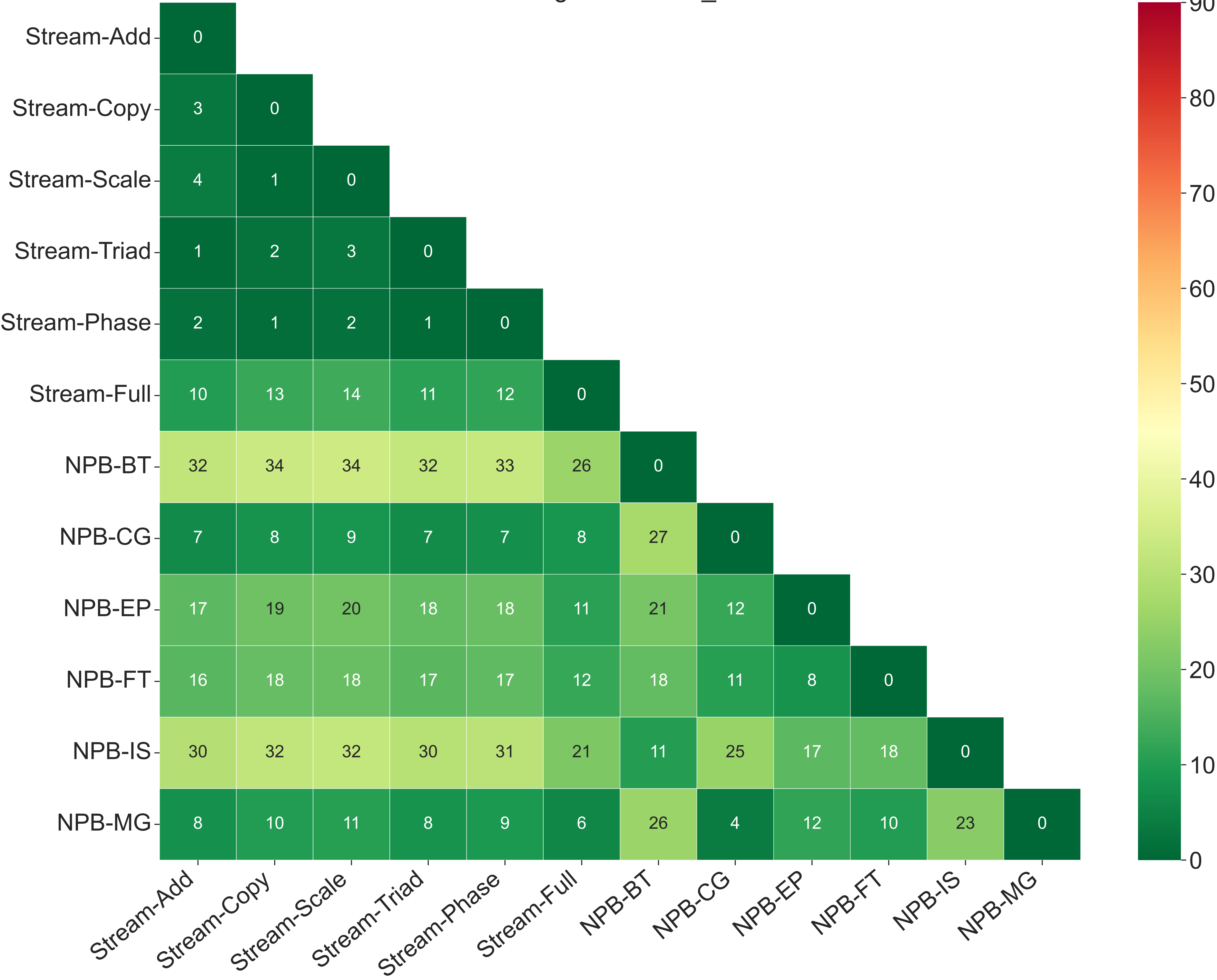
JS-divergence PCAP_107.0
