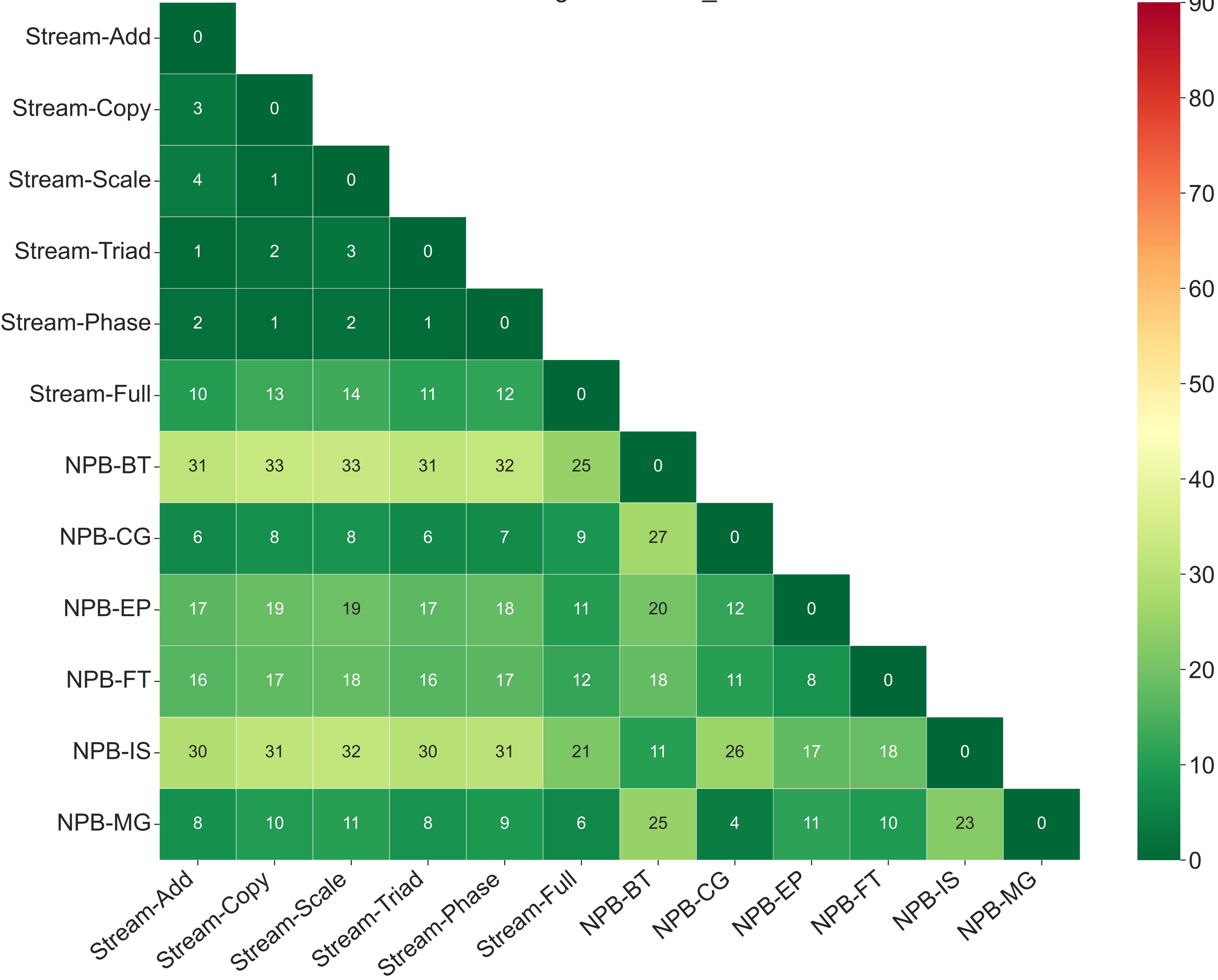
JS-divergence PCAP_118.0
