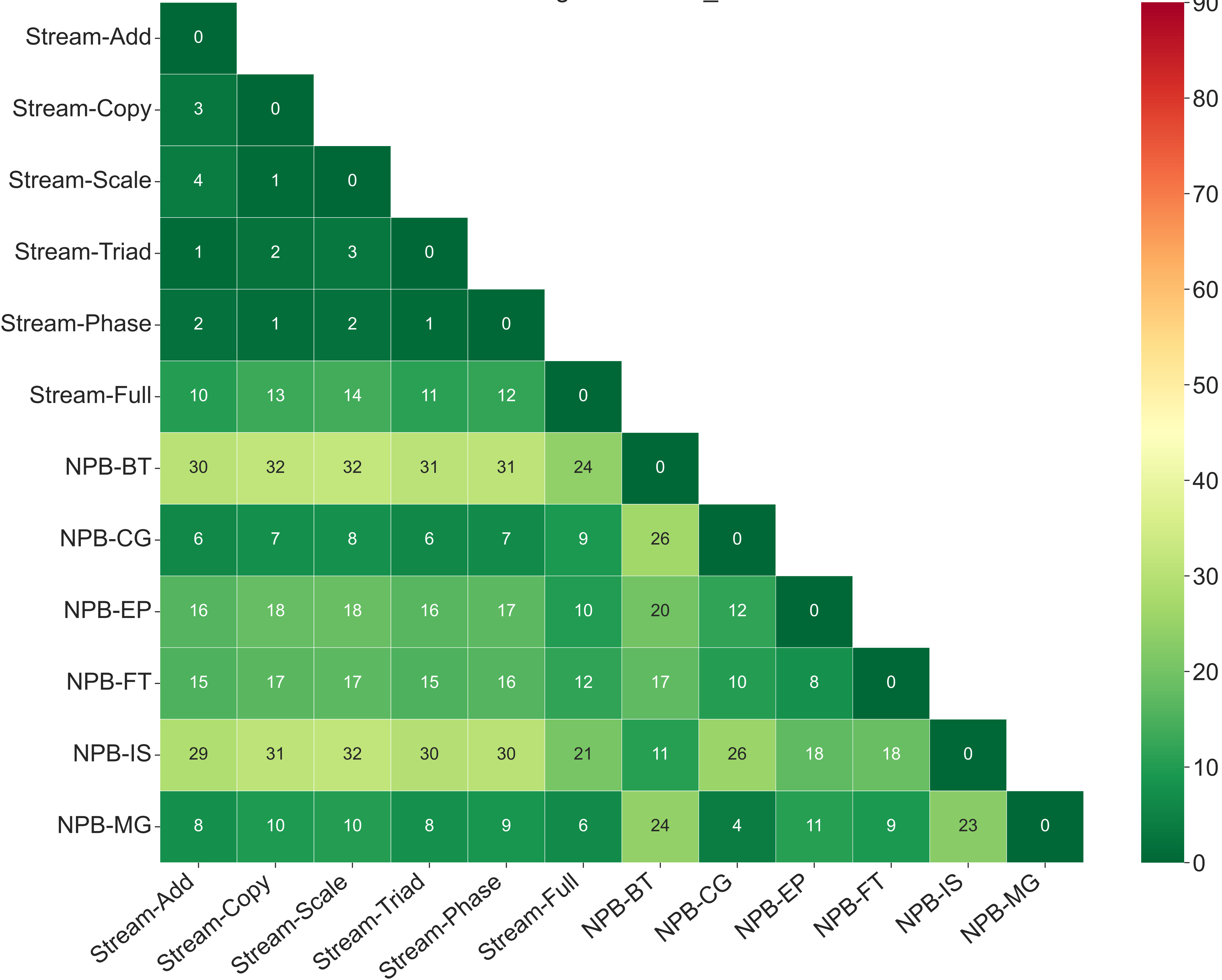
JS-divergence PCAP_136.0
