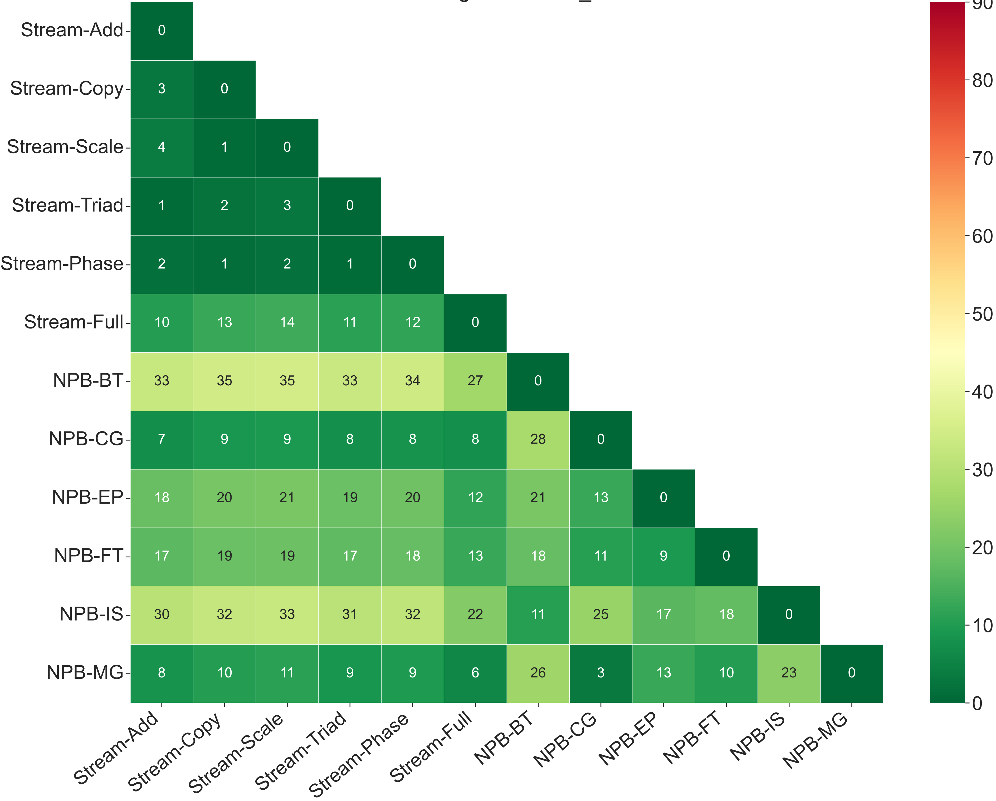
JS-divergence PCAP_95.0
