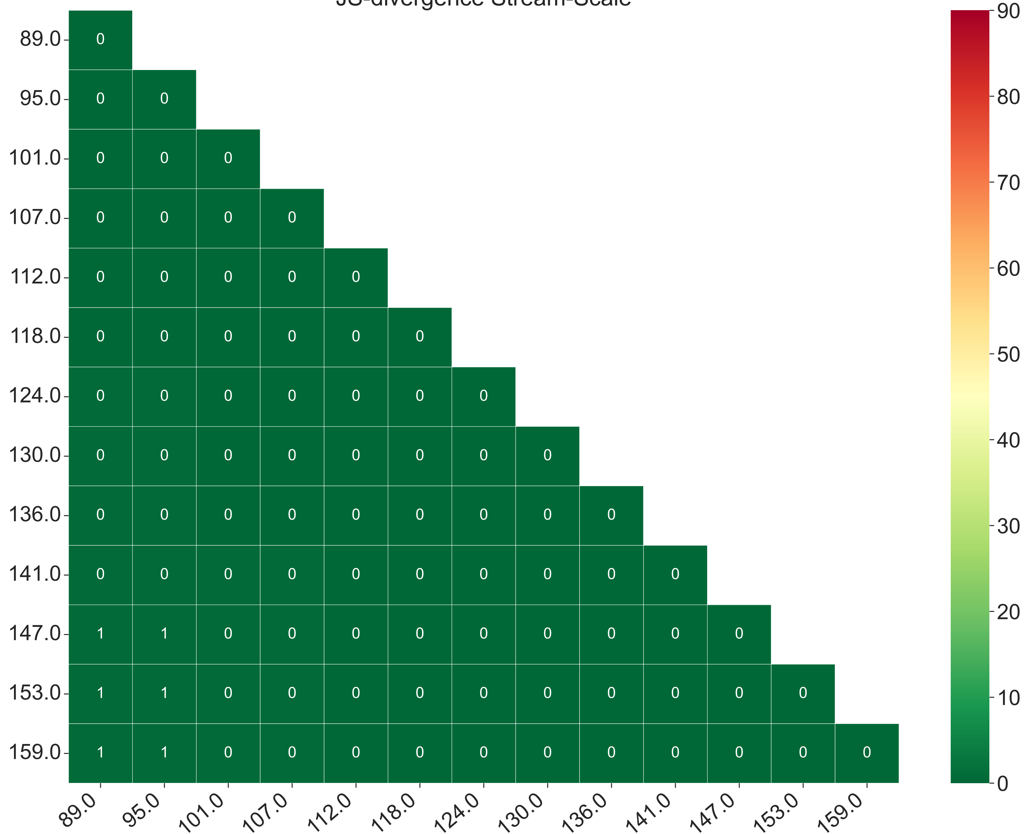
JS-divergence Stream-Scale
