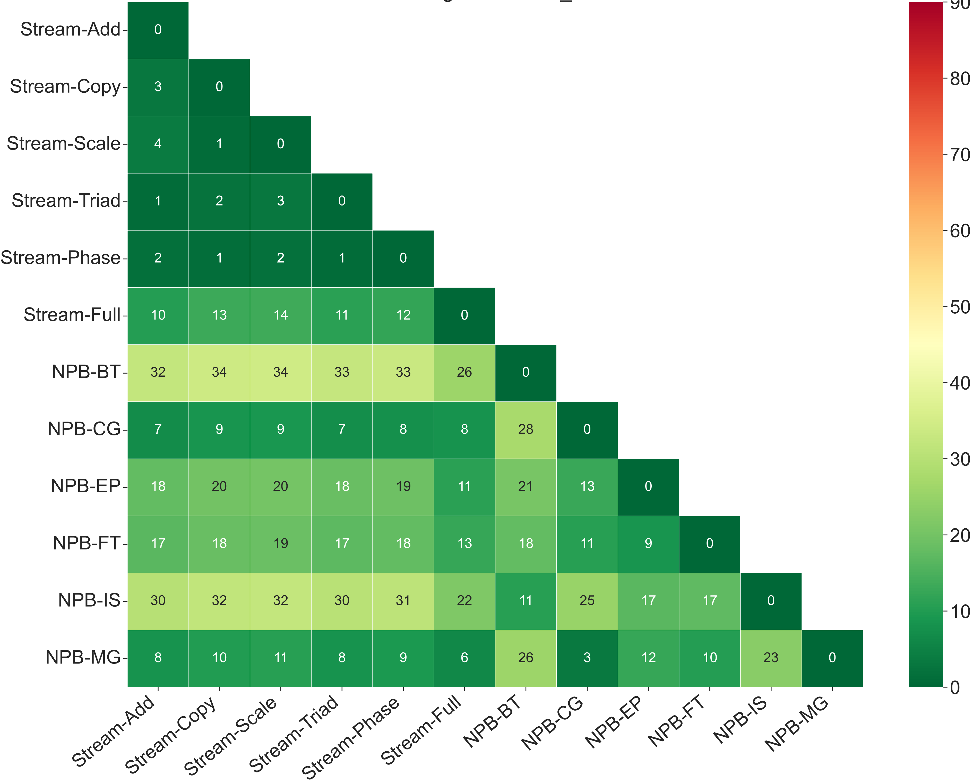
JS-divergence PCAP_101.0
