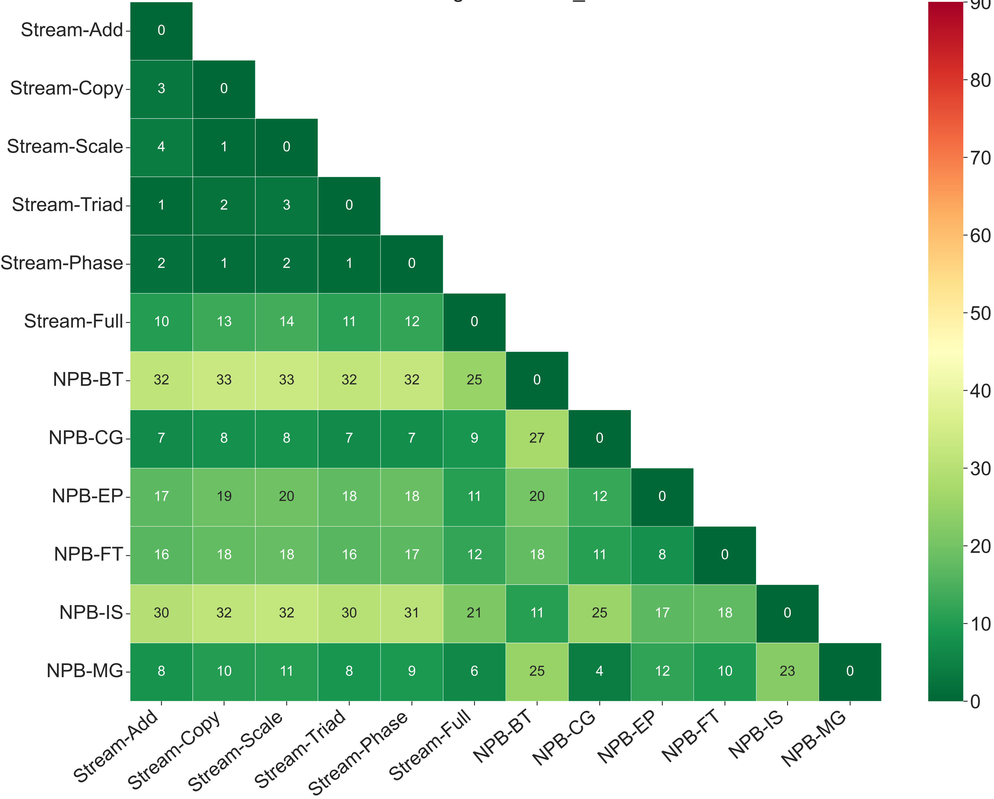
JS-divergence PCAP_112.0
