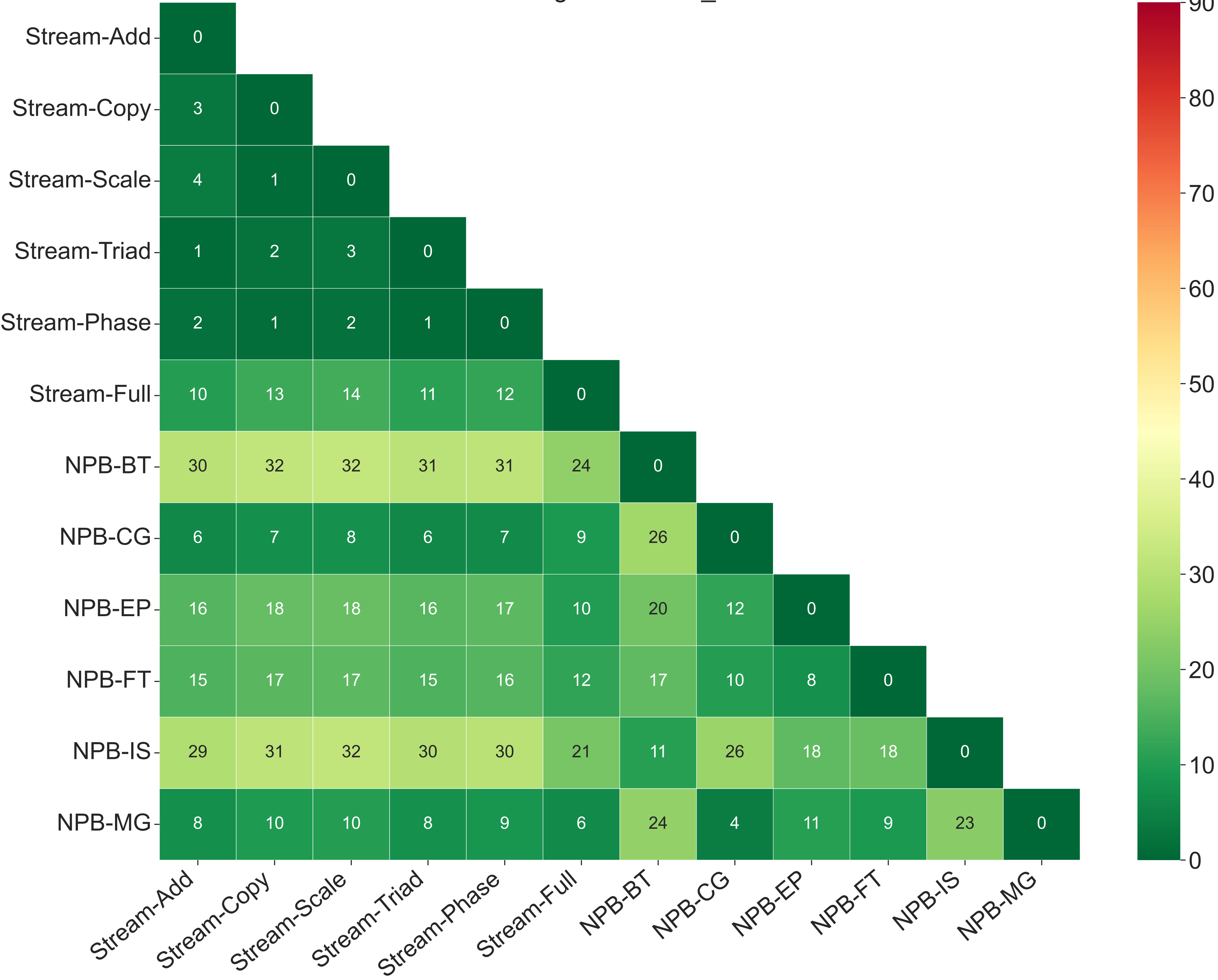
JS-divergence PCAP_136.0
