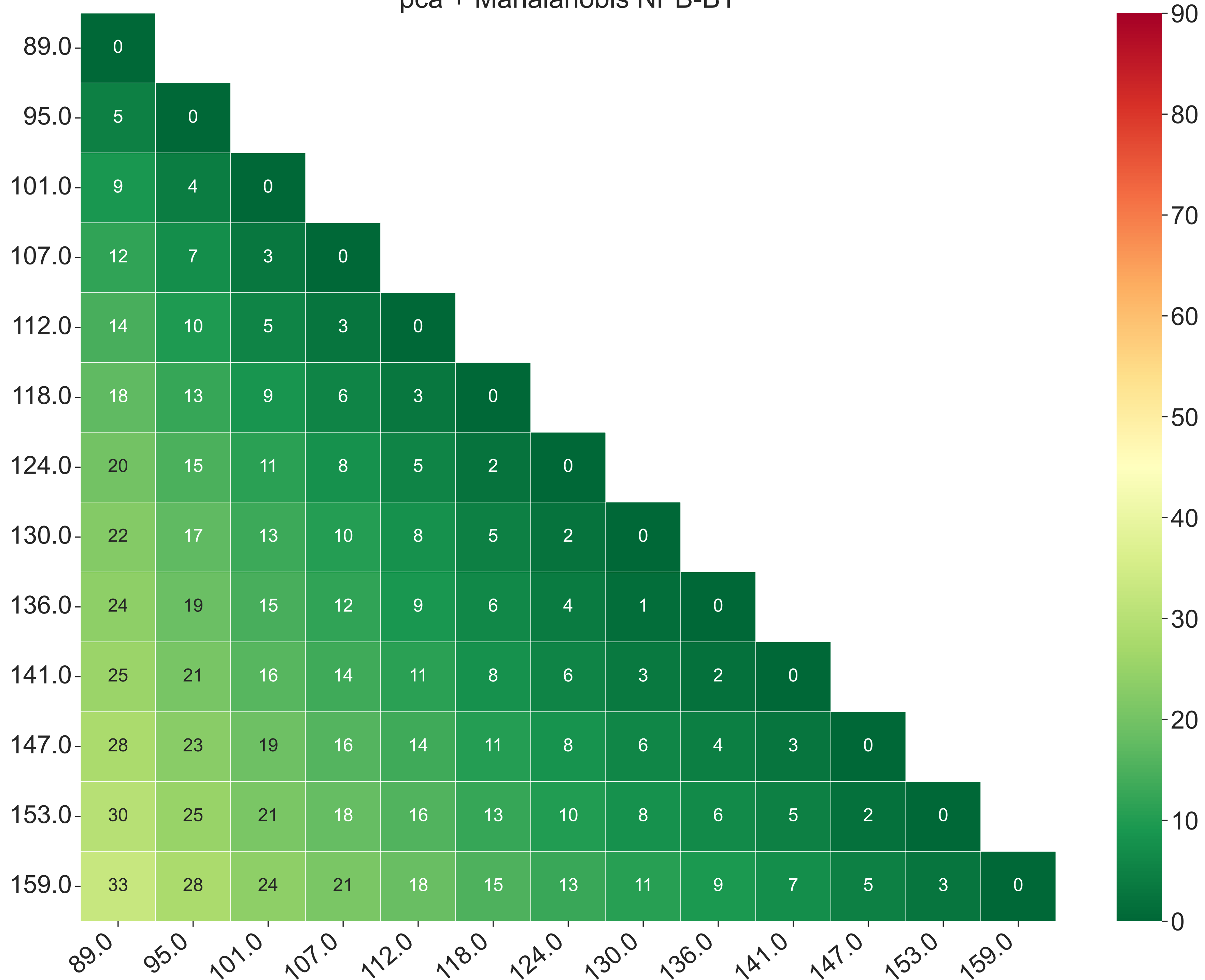
pca + Mahalanobis NPB-BT
