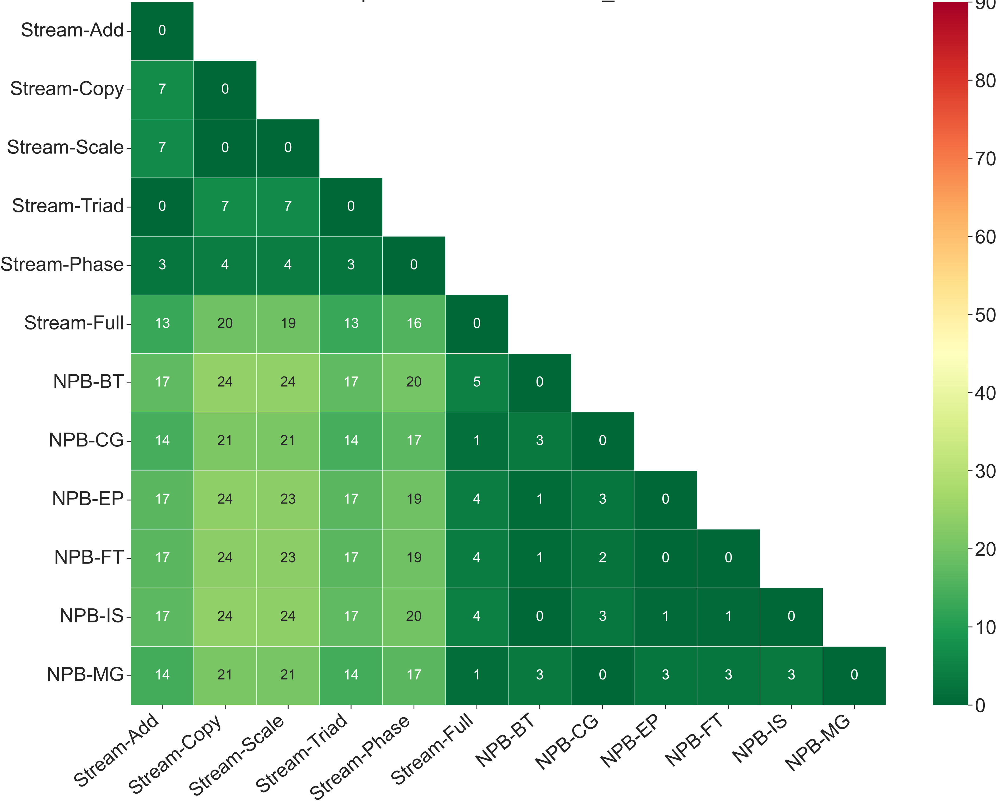
pca + Mahalanobis PCAP_89.0
