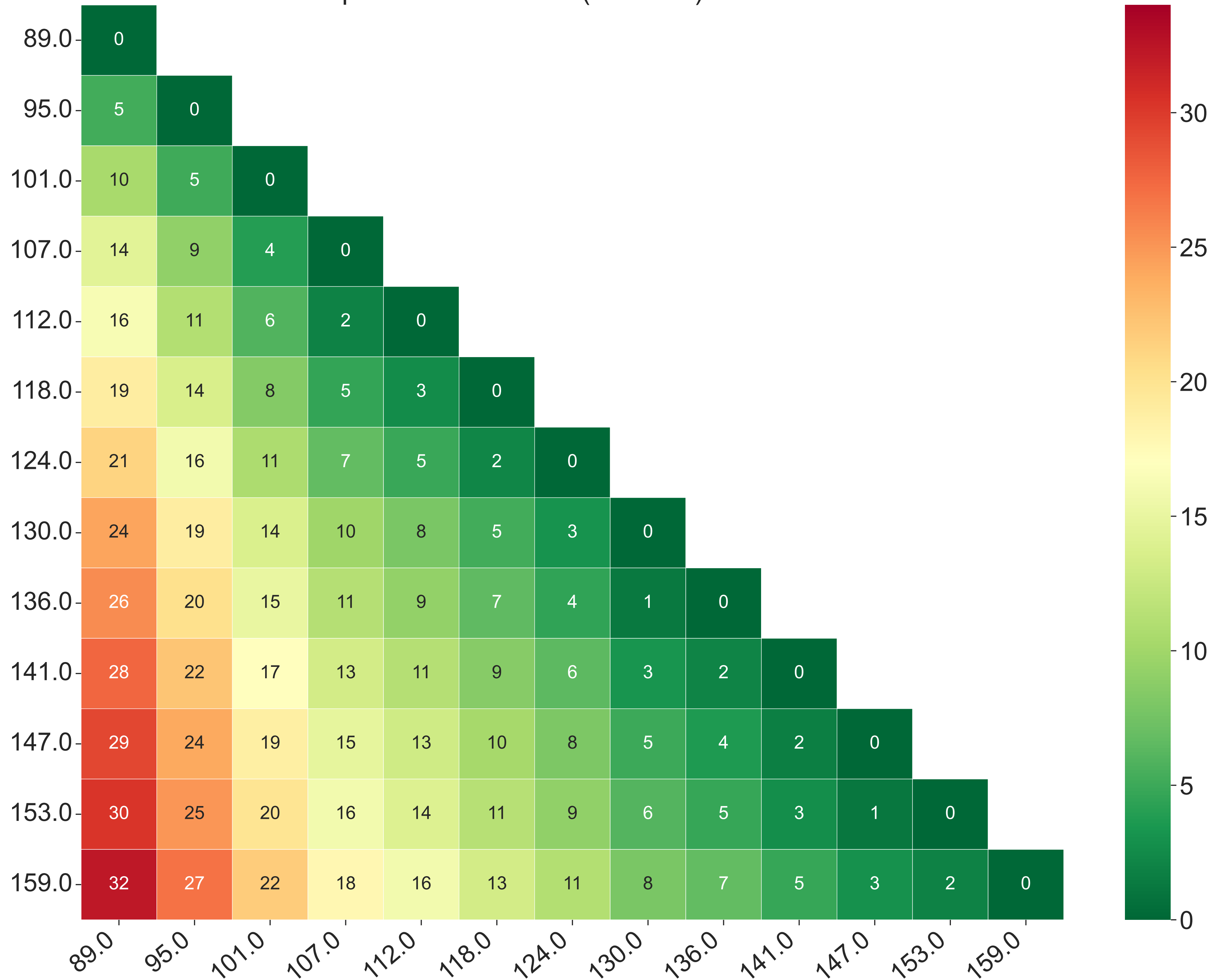
pca + Mahalanobis (rescaled) NPB-IS
