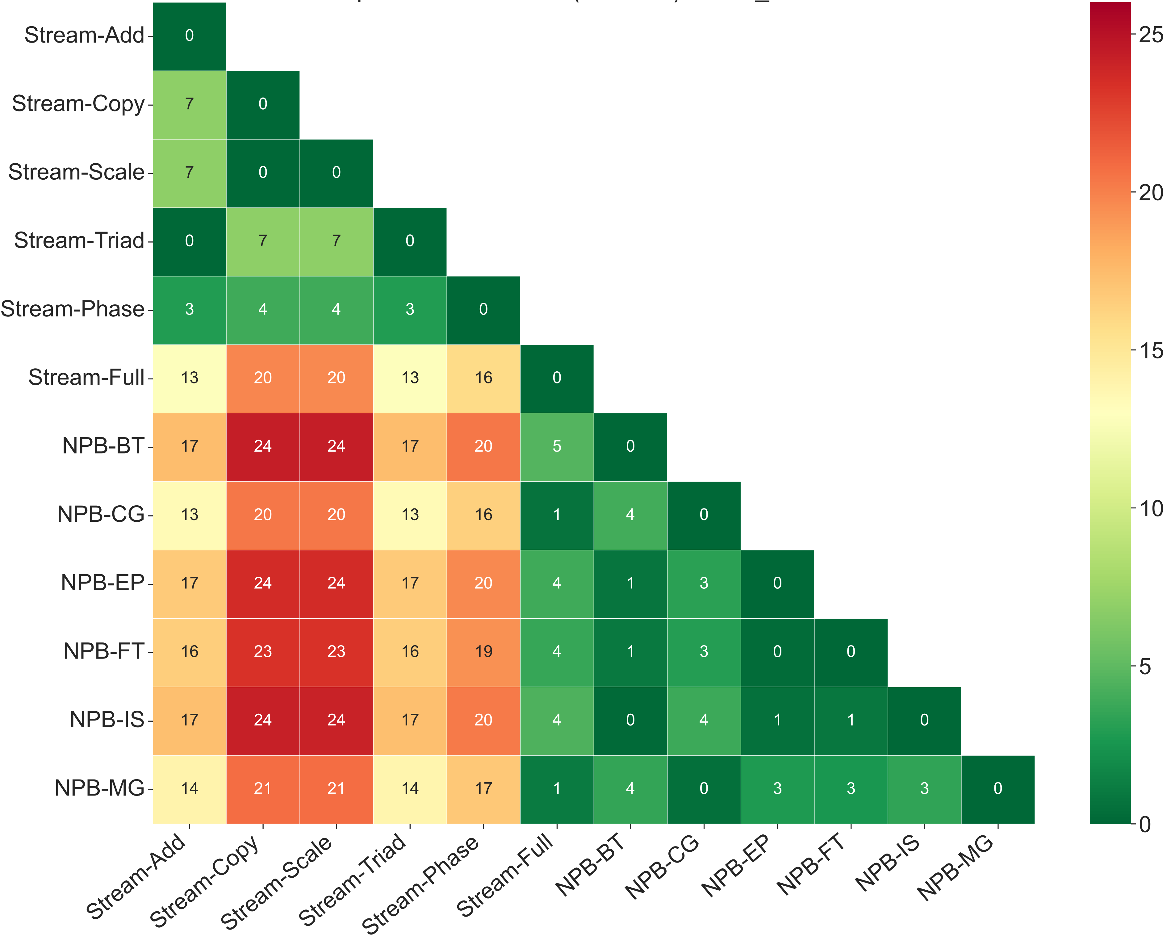
pca + Mahalanobis (rescaled) PCAP_147.0
