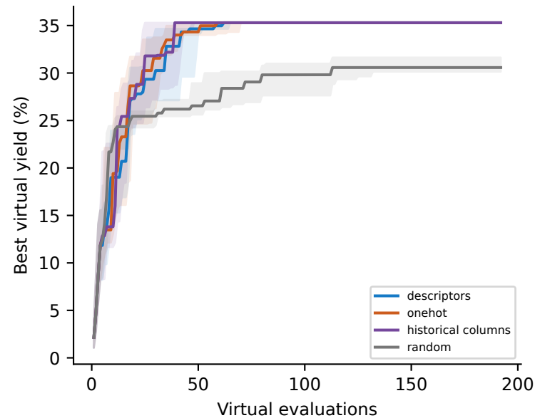
descriptor GP
