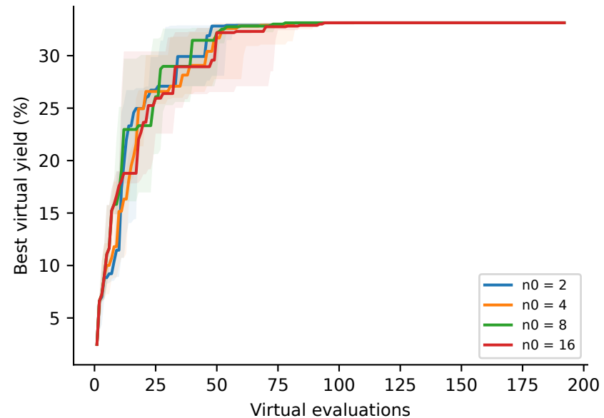
descriptors
