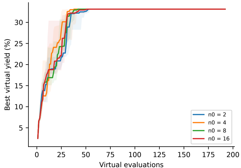
onehot
