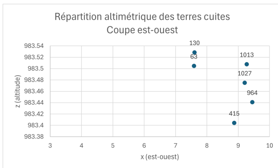
Figure 105. En coupe est-ouest, 964 et 1013 sont des tuiles
