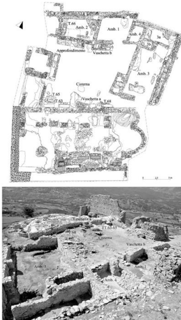
Figure 15. L'organisation spatiale de l'évêché
