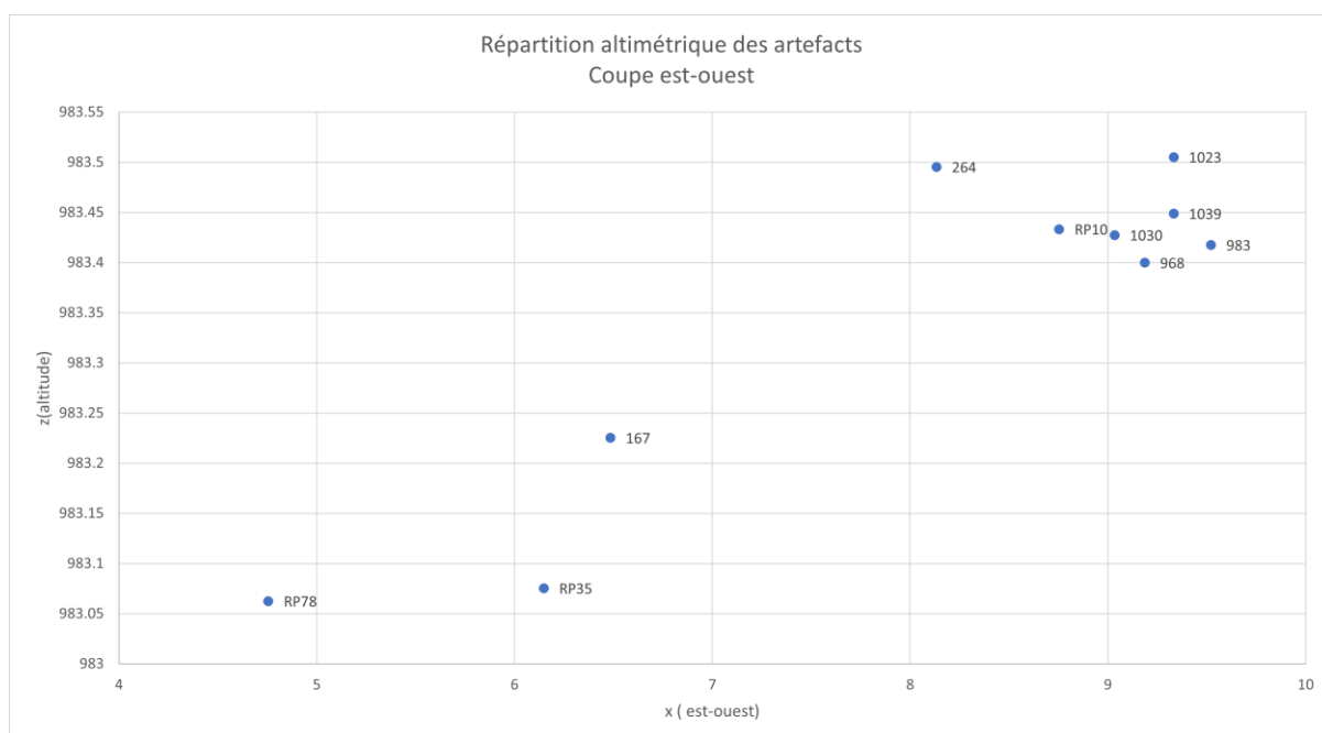
Figure 62. « Métal » coupe est-ouest
