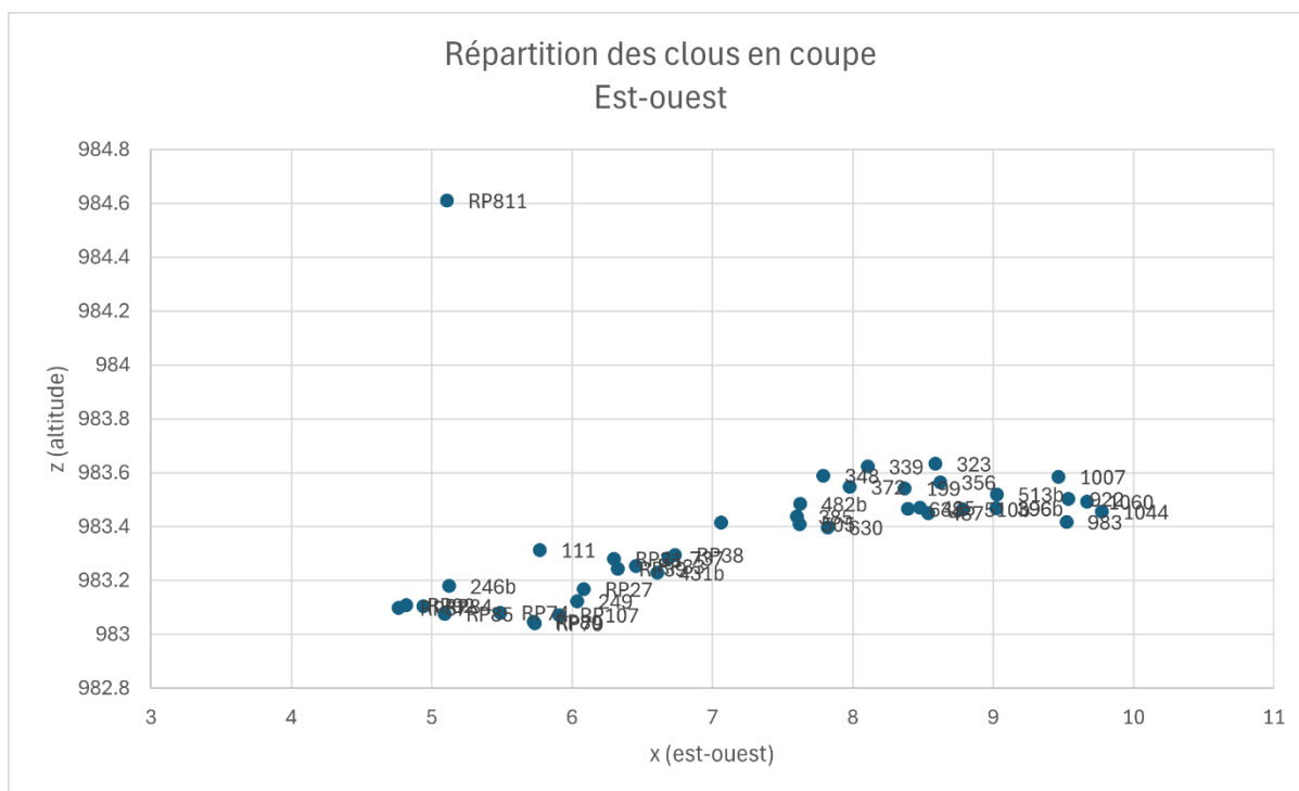
Figure 55. Clous, vue est-ouest
