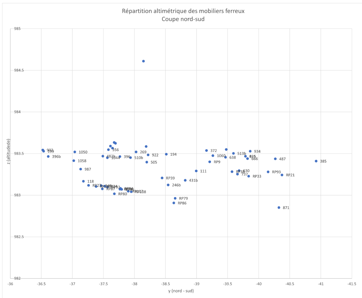
Figure 53. Fer, coupe nord-sud
