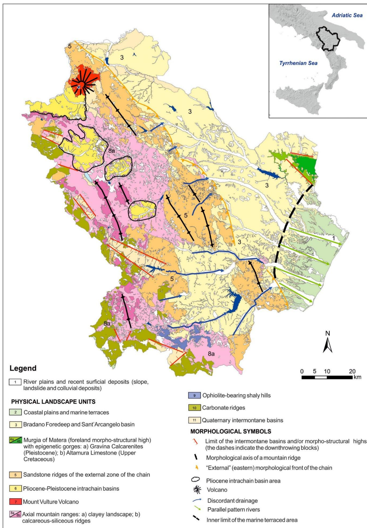
Figure 2. Carte géologique de la Basilicate
