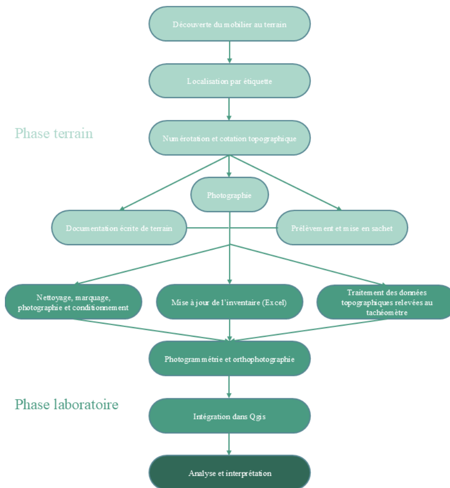
Figure 35. Ordinogramme de la mise en œuvre de la méthode de répartition spatiale
