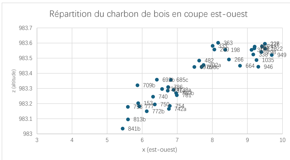
Figure 87. Répartition du charbon de bois en coupe est-ouest
