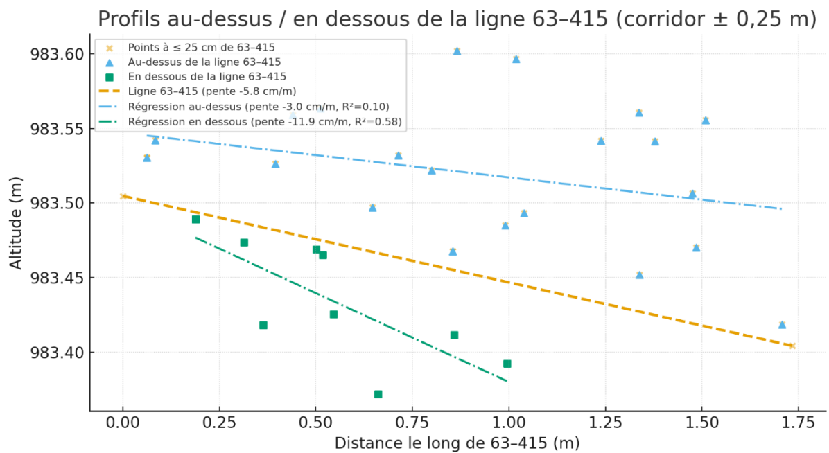
Figure 102. Les pentes dessus et dessous le présumé sol pavé
