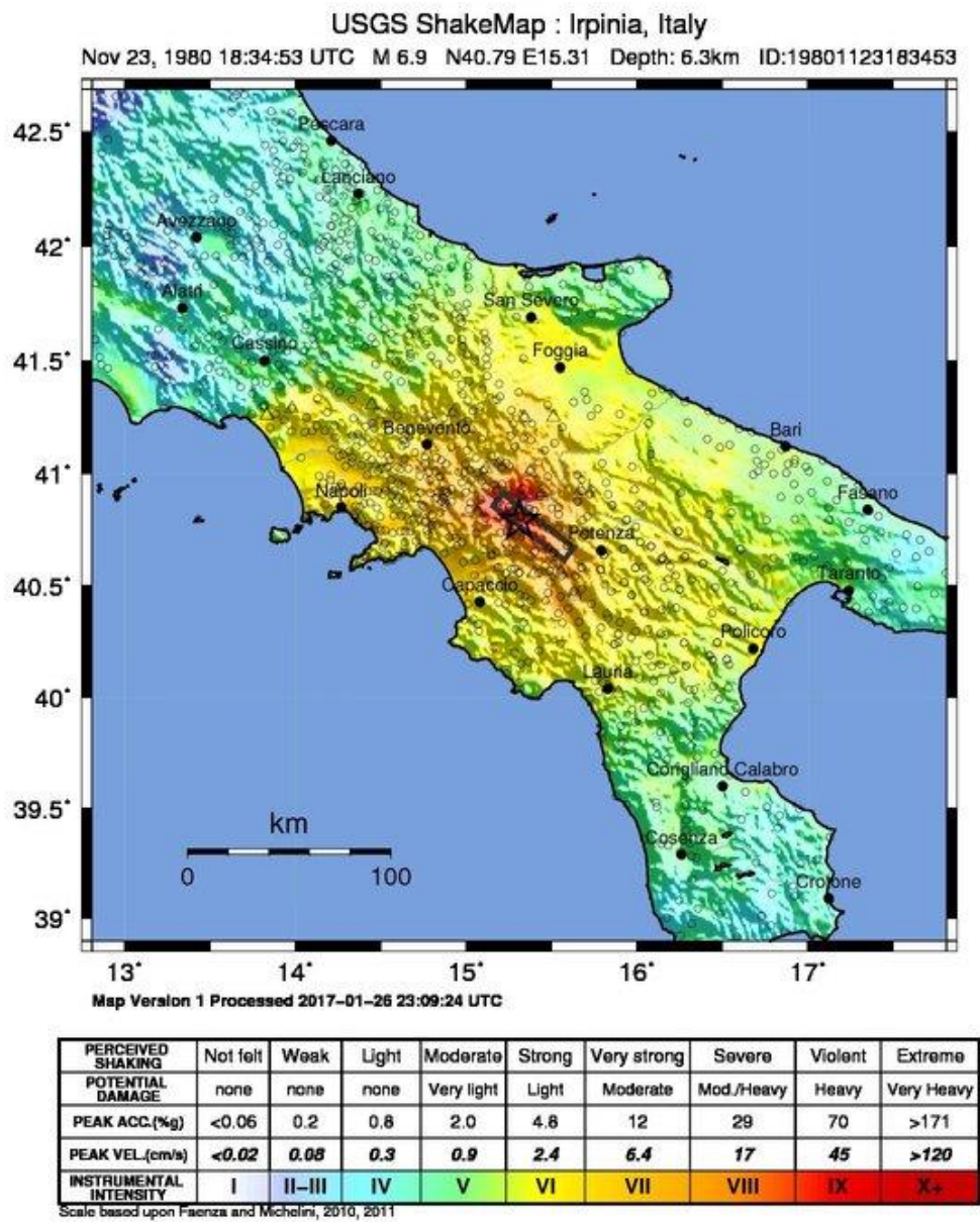
Figure 3. Carte d'impact du séisme d'Irpinia 1980
