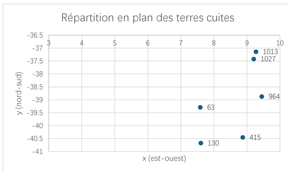
Figure 67. Répartition en plan des terres cuites
