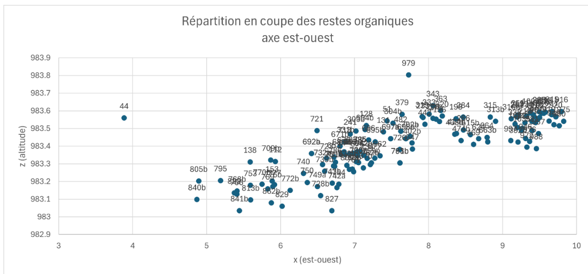
Figure 81. Organiques en axe est-ouest
