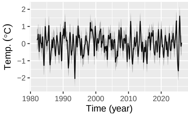
Autoregressive (1)
