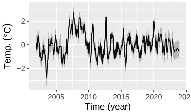
Autoregressive (1)
