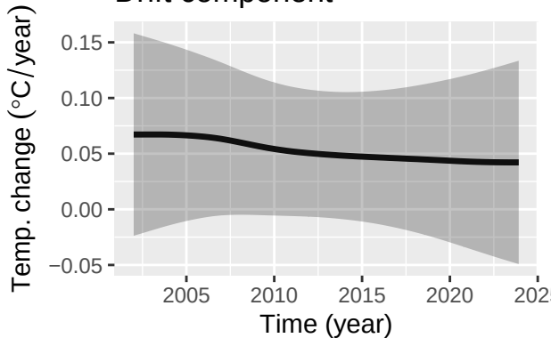
Autoregressive (1)
