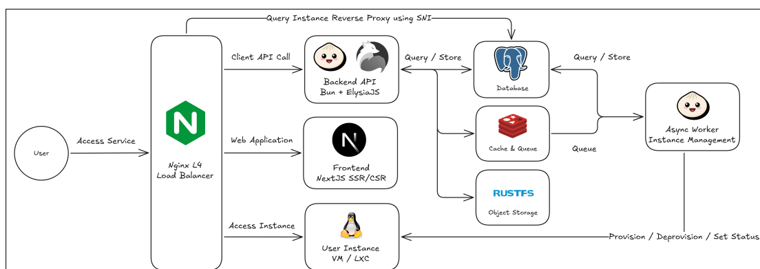
ภาพที่ 4-1 สถาปัตยกรรมระบบโดยรวม
