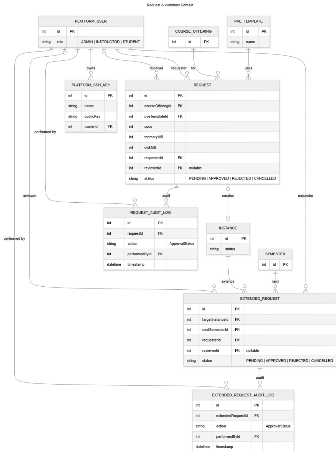
ภาพที่ 3-22 แผนภาพ ER กลุ่มข้อมูลคำร้องขอและกระบวนการอนุมัติ
