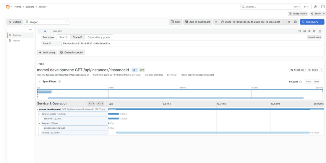
ภาพที่ 4-13 ตัวอย่างผลการติดตามเส้นทางคำขอ (Trace) บน Jaeger
