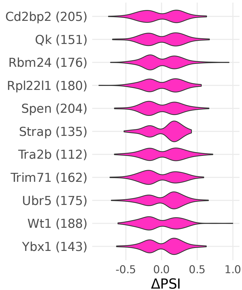
A5SS
