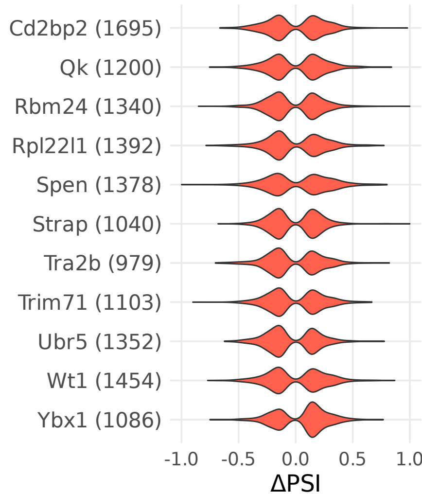
SE
