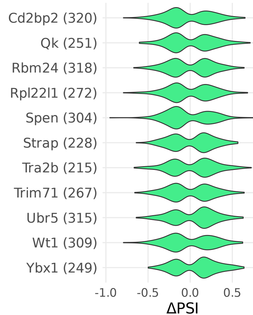
A3SS
