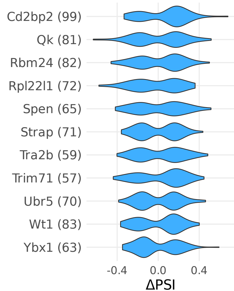
MXE
