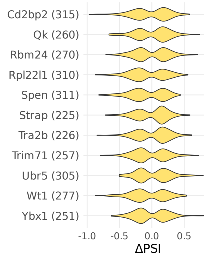
RI
