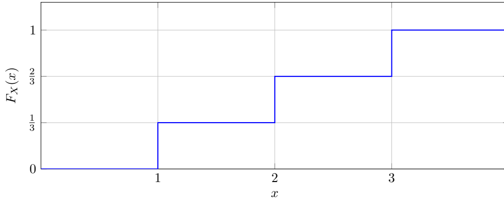
Figura 1: Funzione di Distribuzione Cumulativa per una Variabile Discreta Uniforme su \{1, 2, 3\} .
