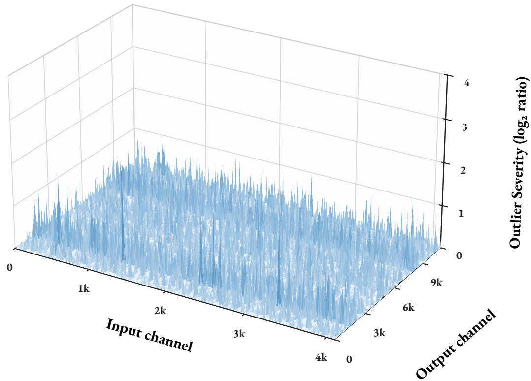
(a) Layer 16 · Weight
