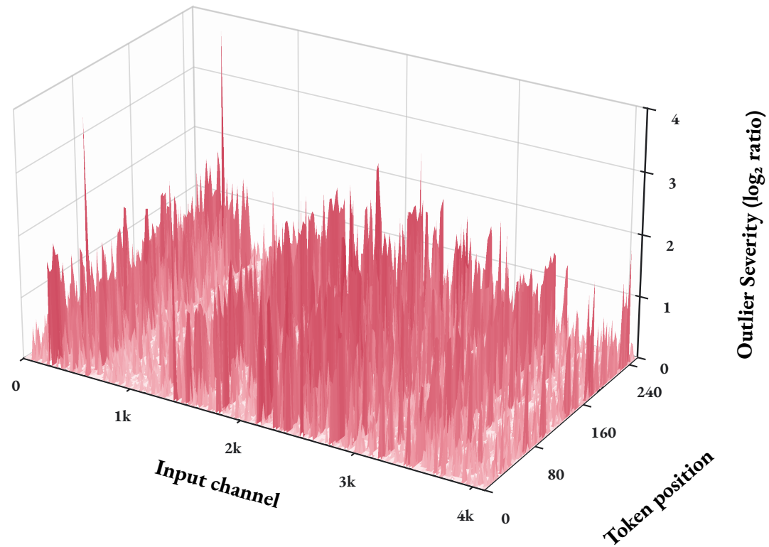
(b) Layer 16 · Activation
