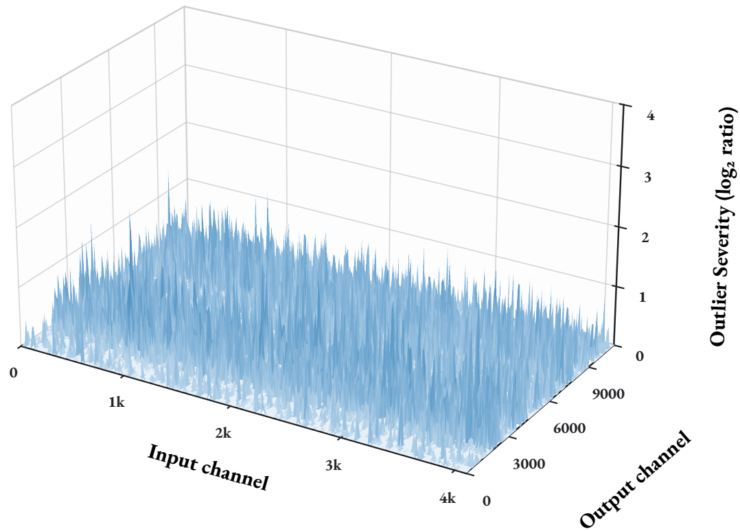
(a) Layer 31 · Weight
