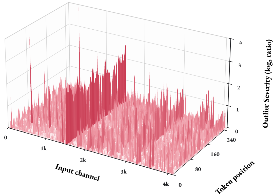
(b) Layer 31 · Activation
