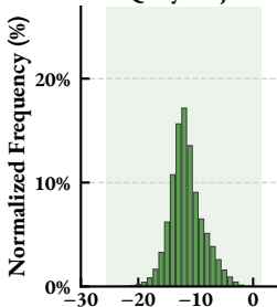
L0: Query Proj.
