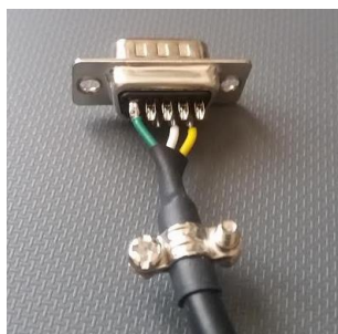
COM1 side (cable male)
