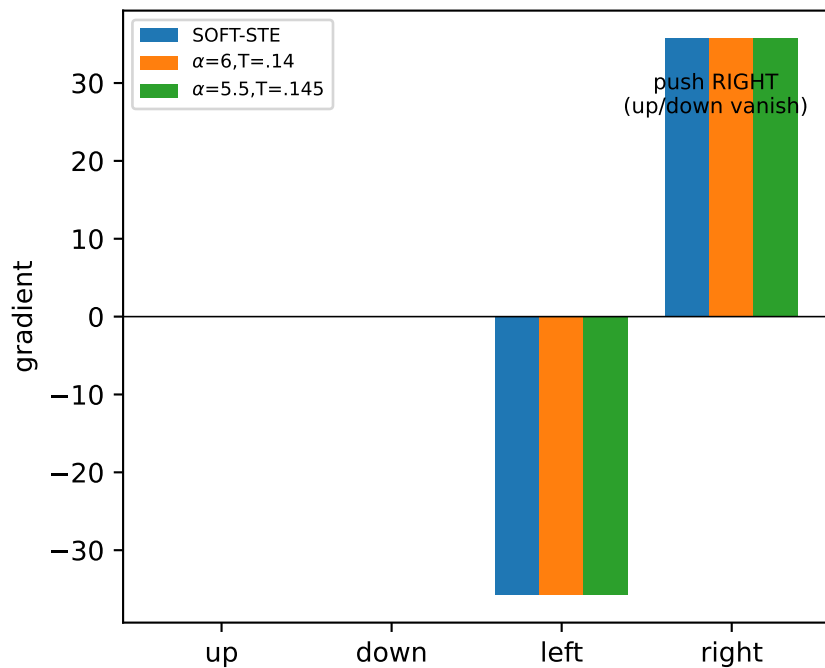
(d) inverse: \partial(\text{move cannon right}) / \partial \text{joystick}
