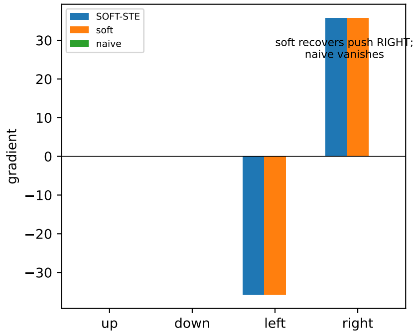
(d) inverse: \partial (\text{move cannon right}) / \partial \text{joystick}
