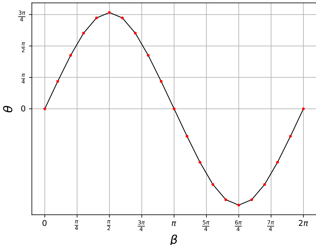
Axion angle vs adiabatic parameter
