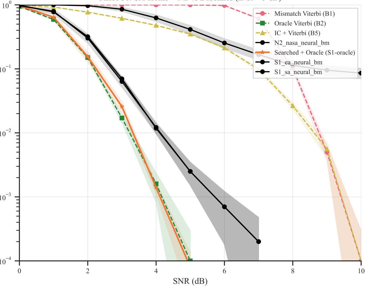
Phase 3c: SA Trellis + N2 vs Baselines (INR = 5 dB)
