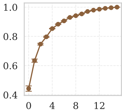
SIFT
