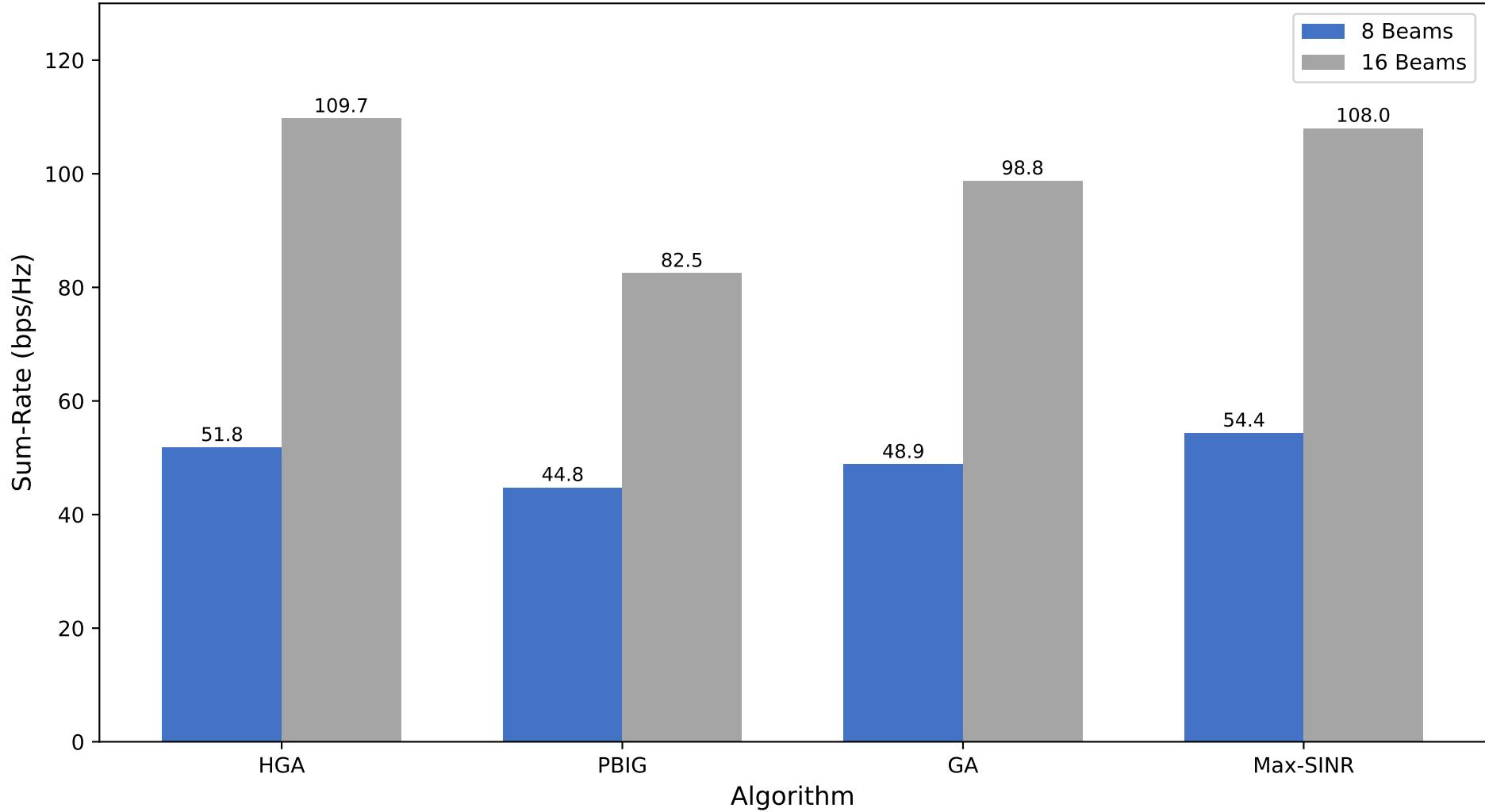
Grafik 6.3: Hücre Başına Hüzme Sayısının Sistem Toplam Veri Hızına Etkisi (40 Kullanıcı)
