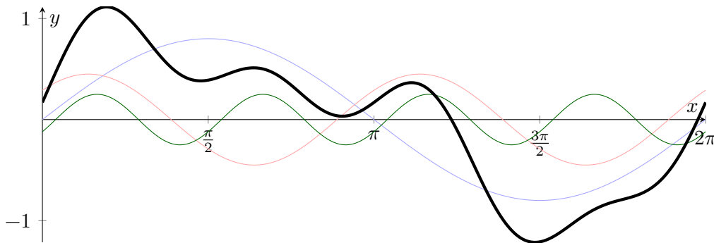
Σχήμα 4: Υπέρθθεση διάφορων ημιτονοειδών κυμάτων.
