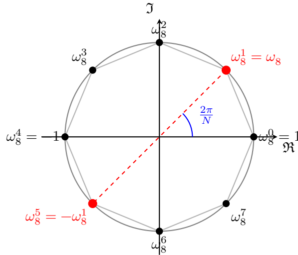
Σχήμα 16: Οι 8-οστές ρίζες της μονάδας στο μιγαδικό επίπεδο ( N = 8 ), σχηματίζοντας κανονικό οκτάγωνο. Η θεμελιώδης ρίζα \omega_8 αντιστοιχεί σε γωνία 2\pi/N (μπλε τόξο). Το αντιδιαμετρικό ζεύγος \omega_8^1, \omega_8^5 (κόκκινο) απεικονίζει τη συμμετρία \omega_N^{k+N/2} = -\omega_N^k .
