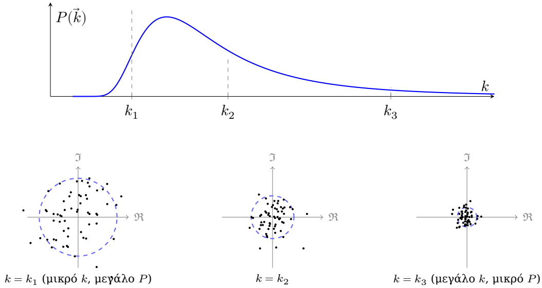
Σχήμα 18: Πάνω: το φάσμα Phillips P(\vec{k}) ορίζει το «περίβλημα» ενέργειας συναρτήσει του k . Κάτω: για κάθε k_i , η τιμή h_0(\vec{k}_i) = \frac{\xi_1 + i\xi_2}{\sqrt{2}} \sqrt{P(\vec{k}_i)} είναι ένα τυχαίο σημείο στο μιγαδικό επίπεδο. Το «σύννεφο» πιθανών τιμών (μαύρες κουκκίδες) έχει τυπική κλίμακα \sqrt{P(\vec{k}_i)} (μπλε διακεκομμένος κύκλος), ενώ η ακριβής θέση μέσα στο σύννεφο καθορίζεται από τις τυχαίες Gaussian μεταβλητές \xi_1, \xi_2 \sim \mathcal{N}(0, 1) . Καθώς αυξάνεται το k , το φάσμα Phillips μικραίνει και το σύννεφο συρρικνώνεται γύρω από το μηδέν — δηλαδή τα κύματα υψηλής συχνότητας (μικρά ripples) έχουν στατιστικά πολύ μικρότερο πλάτος από τα μεγάλα swell waves.
