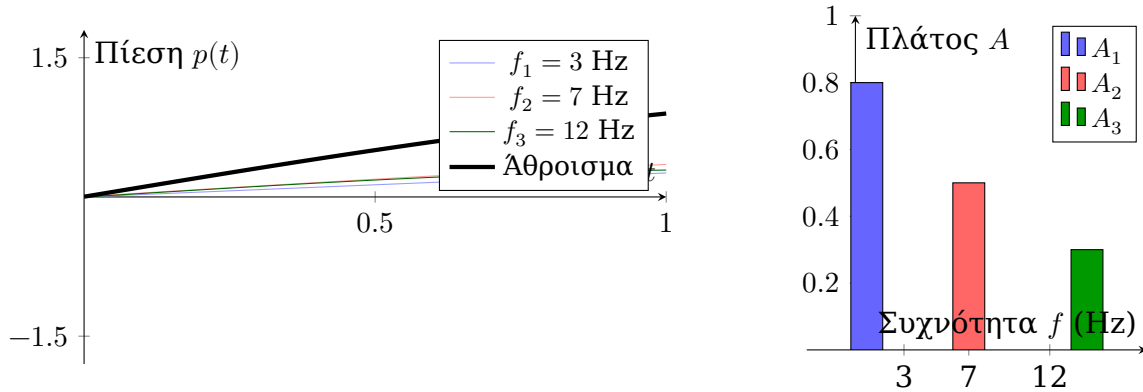
Σχήμα 5: Αριστερά: σύνθετο κύμα (μαύρο) και οι τρεις ημιτονοειδείς συνιστώσες του (αχνά χρώματα). Δεξιά: το φάσμα συχνοτήτων - κάθε ράβδος δείχνει το πλάτος της αντίστοιχης συχνότητας.
