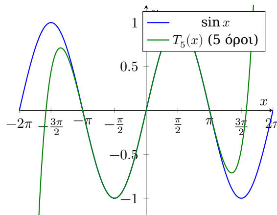
Σχήμα 9: Σύγκριση του \sin x με πολυώνυμο Taylor 5 όρων.
