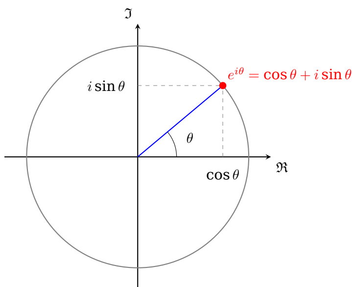
Σχήμα 11: Μιγαδικό επίπεδο: η γραφική αναπαράσταση του τύπου του Euler.
