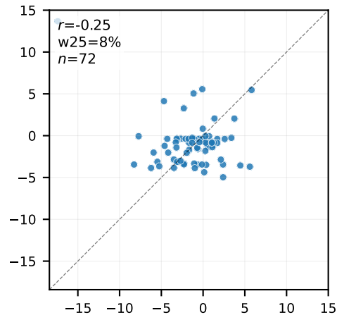
Sonnet 4.6
