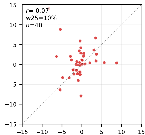
GPT-5.4
