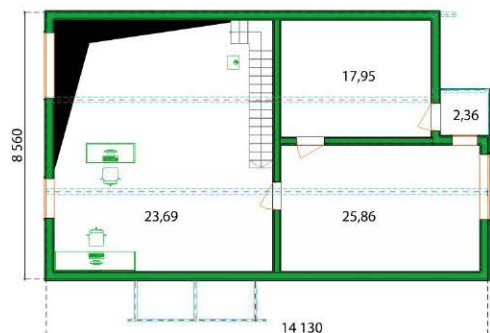
План 2 этажа
