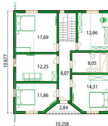
План 2 этажа
