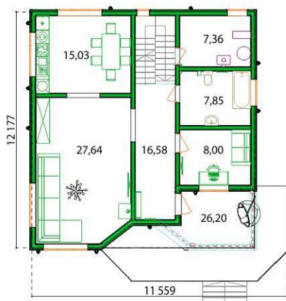
План 1 этажа
