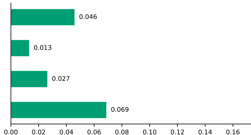
gemma-4-E4B-it
