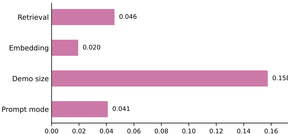
gemma-4-26B-A4B-it
