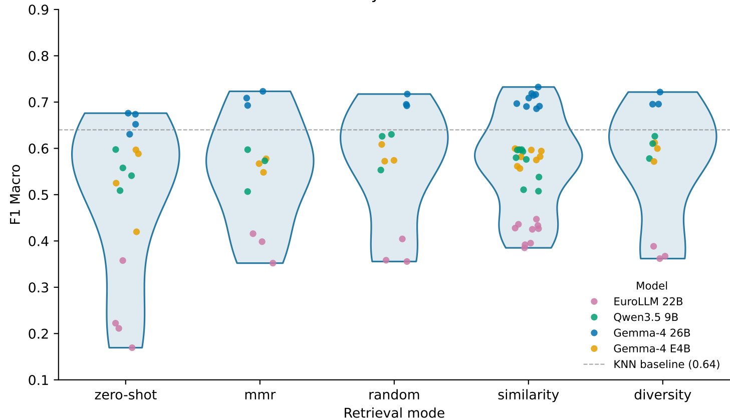
F1 Macro by Retrieval Mode
