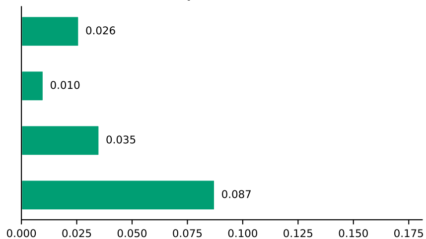
gemma-4-E4B-it
