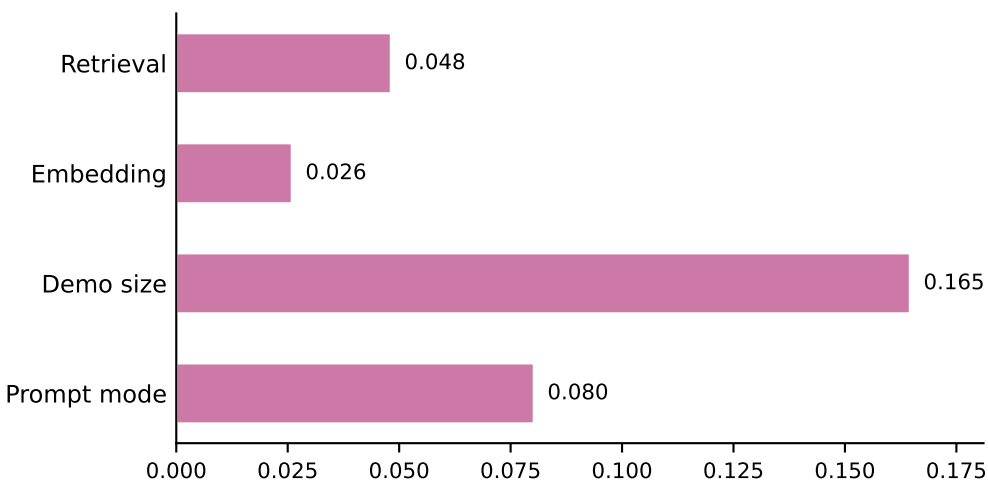
gemma-4-26B-A4B-it
