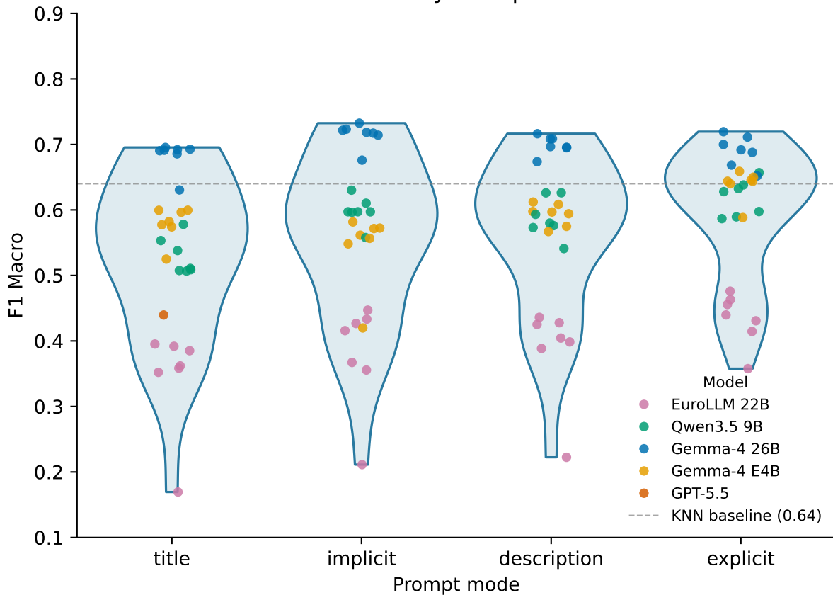
F1 Macro by Prompt Mode
