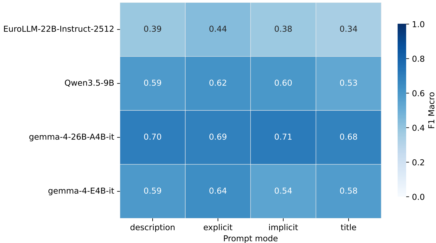
Mean F1 Macro — Model × Prompt mode
