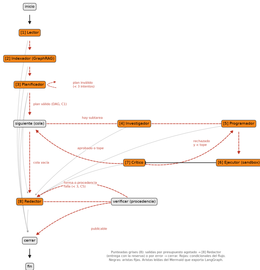
Ilustración 4. Diagrama del orquestador (LangGraph) con sus aristas condicionales
