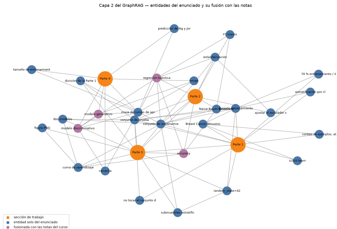
Ilustración 6. Capa 2 de la Tarea A: entidades del enunciado fusionadas con las notas del curso
