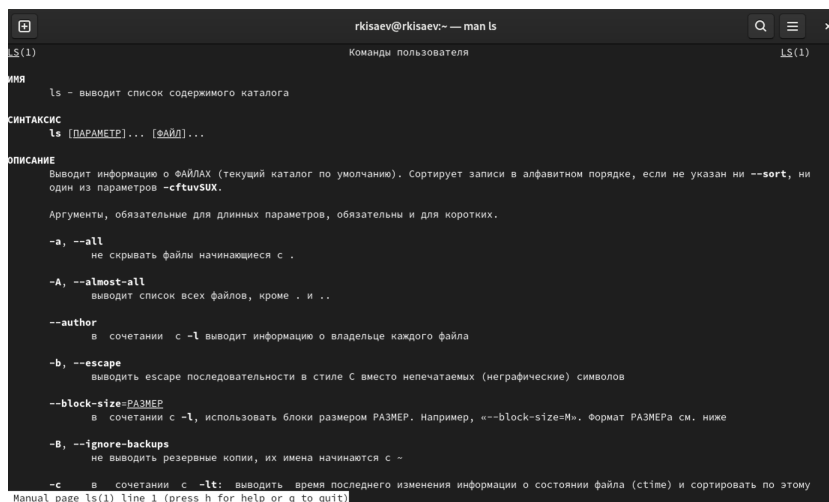
Рис. 4.11: man ls
