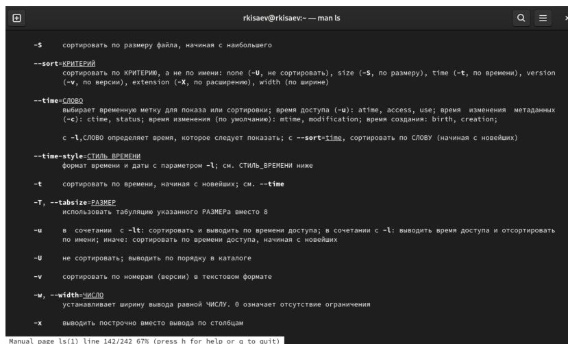
Рис. 4.12: time style
