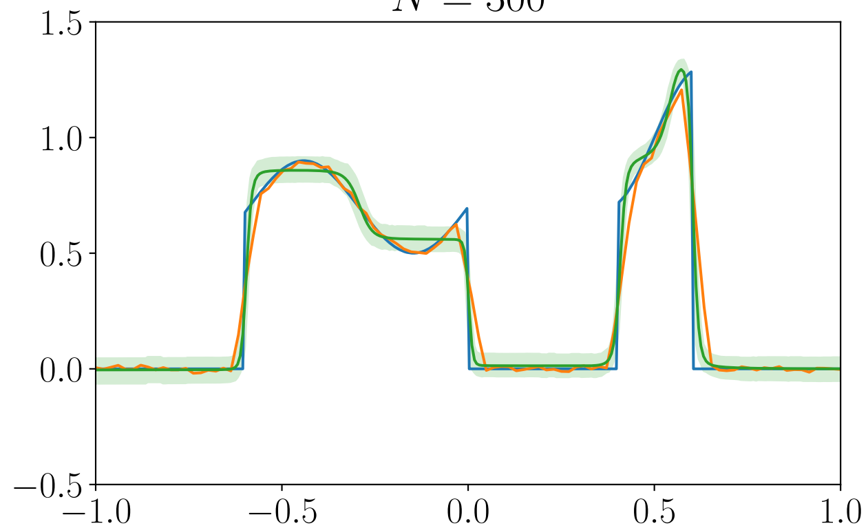
N = 300
