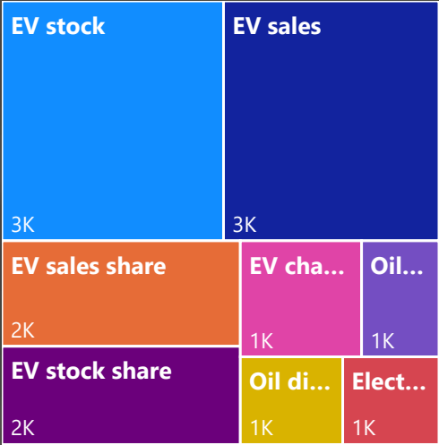
Parameter Count
