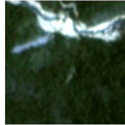
RGB tile 296
