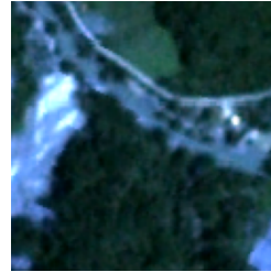
RGB tile 221
