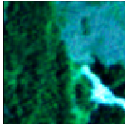
RGB tile 30
