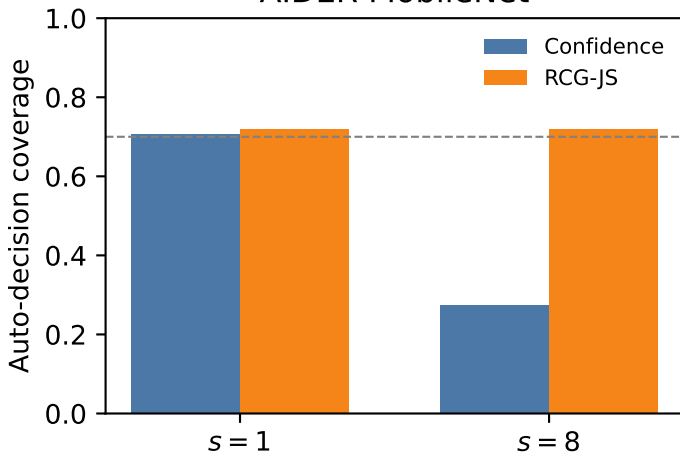
AIDER MobileNet
