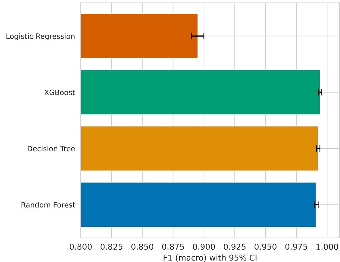
UGRansome2024
