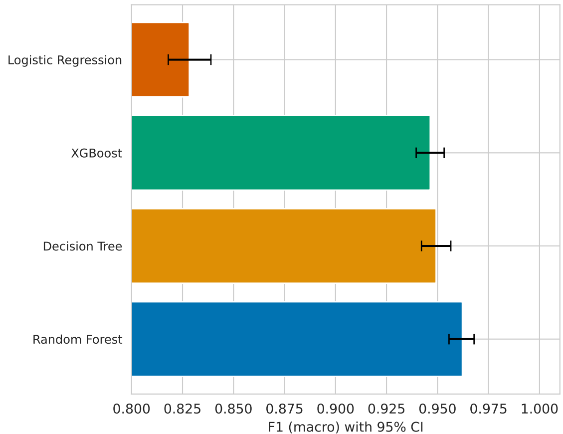
CICIoT2023
