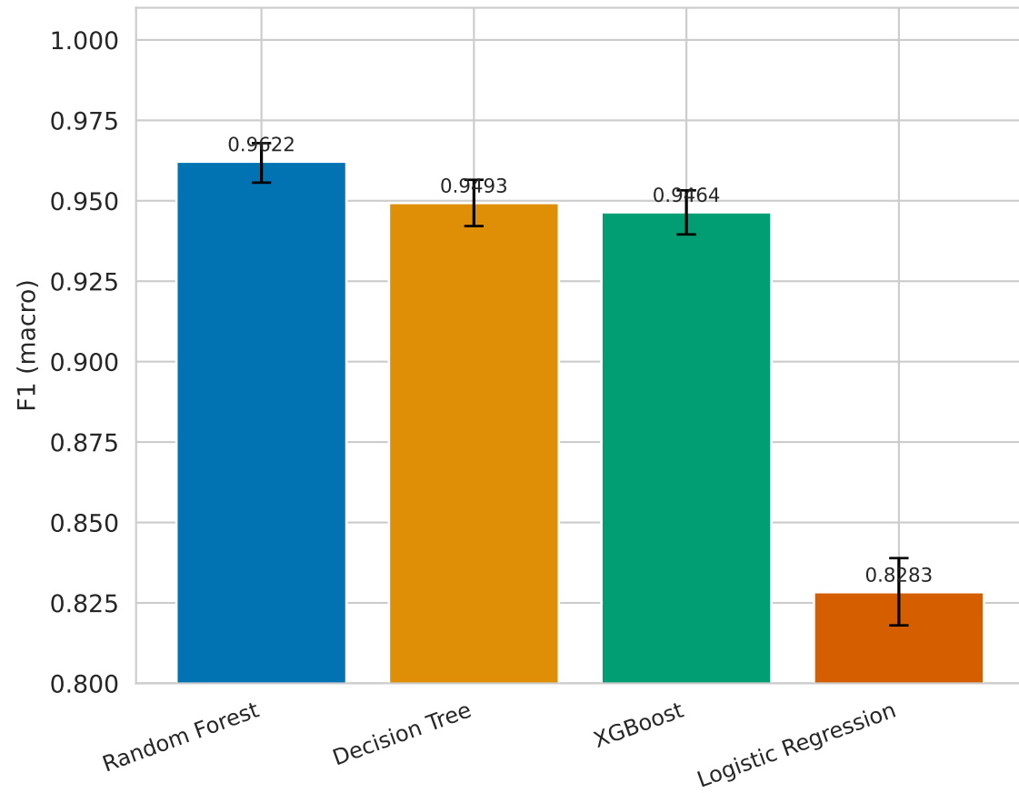
CICIoT2023
