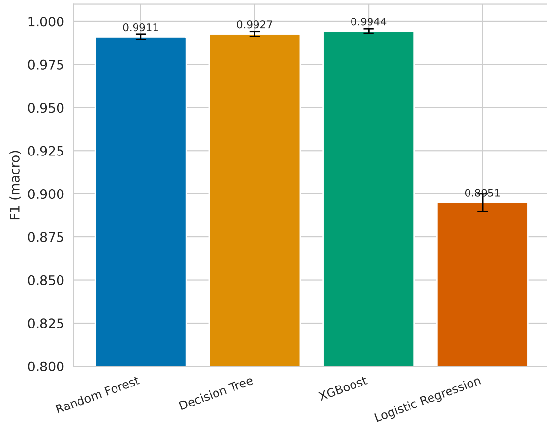
UGRansome2024
